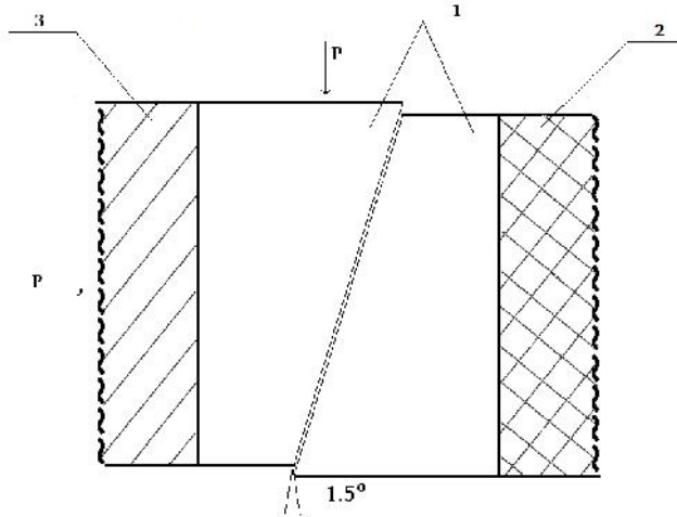
ნახ.№2. შეუღლებული კონუსების წყვილი. 1 -კონუსების წყვილი; 2 - დამჭერი რგოლის კედელი; 3 - წნეხფორმის კედელი.
