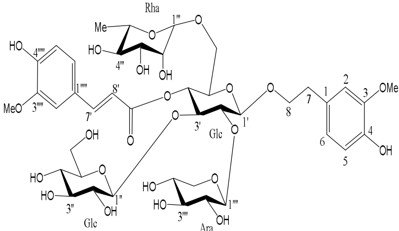
ფერუგოზიდი A
