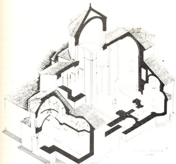
ტაბრის აქსონომეტრიული ნახაზი.
