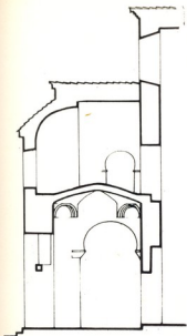
გრძივი კვეთი კარიბჭეზე, ხელი ჩაღლირებისაკენ.
