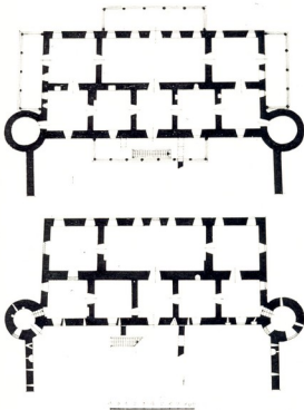
ლამისკანის სასახლე. I და II სართულის გეგმა რესტავრაციის შემდეგ.
