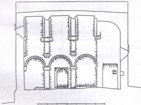
სურ. 5. სათლეს ეკლესიის სამხრეთი ნაწილი.
