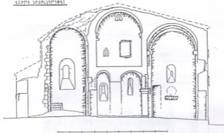
სურ.4. საილეს ეკლესია. განივი ჭრილი.
