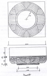
სურ.1. საირხის კაპიტელი. გრაფიკული წარმართვა.
