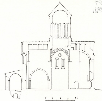
Бетания. Разрез.
