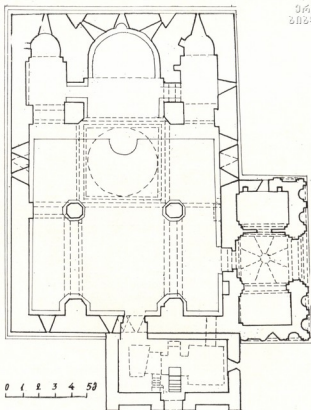
ბეთანის ტაძრის გეგმა.
