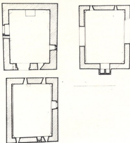
კოშკურა საცხოვრებელი. გეგმა.
