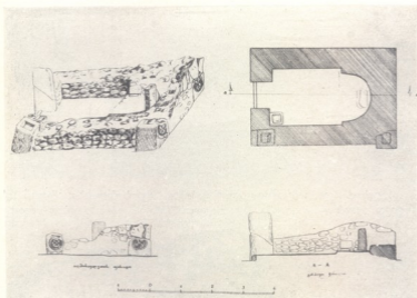
მცირე ეკლესია მდ. კაზრეთულას ფერდობზე, გეგმა და კრილები
