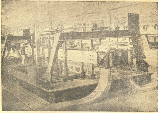
დნებრის ალიუმის კომბინატი. — აპაზა ნა, რომელშიაც ხდება ალიუმის მიღება.
