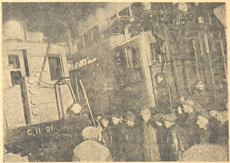
პირველი საბჭოთა შედუღებული ორთქლმანაუსი, ამ 114 ტონიანი ელექტრომაგვლის პროექტი შედგენილია საბჭოთა სპეციალისტების მიერ და 8 თვის განმავლობაში იქნა აგებული ქარხანა „დინამო“-ს (მოსკოვი) მუშებისა და იმპერეტენიკოსების დაუღალავი მუშაობის წალობით საბჭოთა მახალბიდან. ელექტრომაგვლების მშენებლობის ორგანიზაცია წარმოადგენს უდიდეს ნაბიჯს საბჭოთა ქვეყნის ეკონომიური დამოუკიდებლობის გზაზე და თითოეულ ელექტრომაგვლზე გვიწოვავს 800.000 მანეთს ოქროთი. სურათზე—ელექტრომაგვლის გამოცდა.
