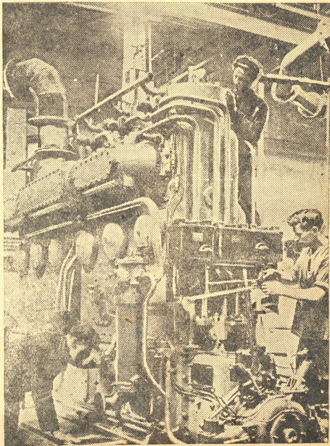
წულტერის ახალი სისტემის 1800 ცხ. ძ. დიზეილი, რომელსაც ამზადებს...
