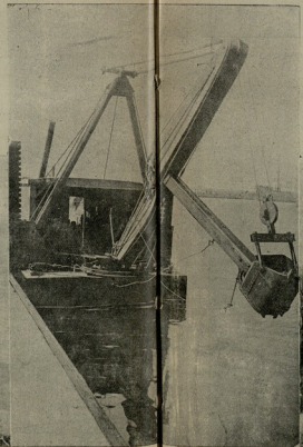
მიწის მოხრელი და ამწევი რაკობის საშუალებითაც
