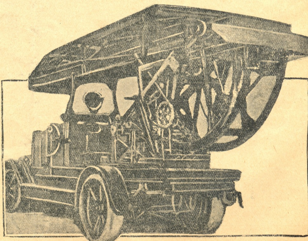
ახალი ციკლსაქმობა კიხე, დამზადებული, ხარკოვის ციკლის მქორბოელი რაზმის მექანიკოს ლაკაზის მიერ. კიხის სიმაღლე 24 მეტრს უდრის, ღირს 8.500 მანეთი. უტახეთში დამზადებული ამგვარი კიხე 30.000 მანეთი ღირს.
