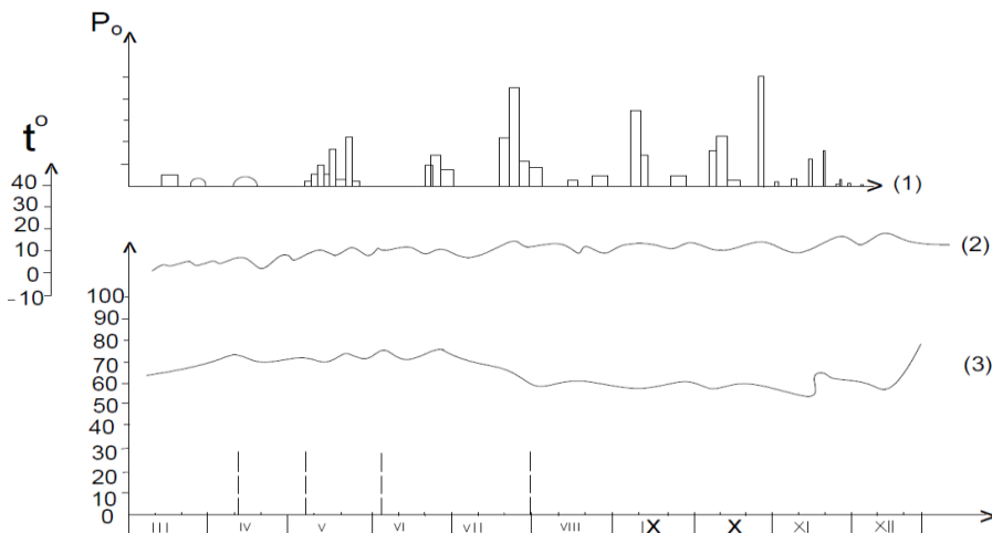
ნახ. 1. ატმოსფერული ნალექები (1), ჰაერის ტემპერატურის (2) და ნიადაგის ტენიანობის (3) ცვალებადობის გრაფიკები
