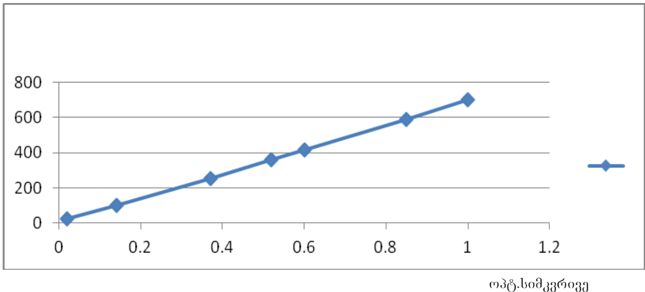
ნახ.1. ცილის საკალიბრო მრუდი (ბრედფორდის მეთოდით)
