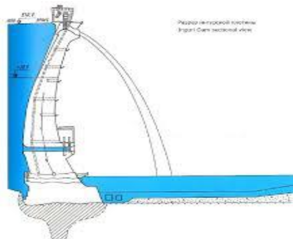
Рис.2 Схема плотины
