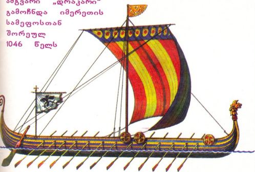
საბრძოლო ნავი „ლიდა“ რომლითაც რუსებმა კასპის ზღვისა და მტკვარზე დაშტრობდნენ
