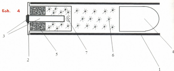
1 - ლულა; 2 - მასრა; 3 - ფისტონი; 4 - ტყვია; 5 - დენთის დაუმწვარი ნაწილაკე-ბი; 6 - დენთის ცეცხლოკიდ-ბული ნაწილაკეები; 7 - ფის-ტონის აფეთქების ალი.
