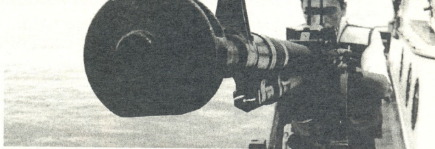
ჩვენი დროსი: „გენერალი მახნიაშვილი“ ორი ტყვიამფრქვევითაა შეიარაღებული, მათგან ერთი 12,788 კალიბრის საზენიტო ДАК-ი. 9-კაციანი ეკიპაჟის საშტაბო შეიარაღებაშია მოკვლეულიანი „კალაშნიკოვები“, ხელის ტყვიამფრქვევი და ტანკსანიანაღმდეგო ყუმბარსატყორცნი.
