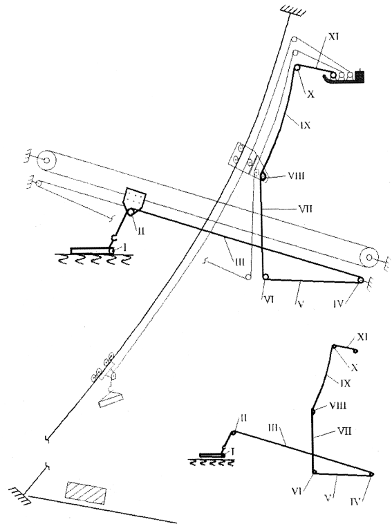
ნახ. 1. ა, ბ — განივადსატანი ჩაკეტილკონტურიანი ბაგირ-ბლოკური საბაგრო
