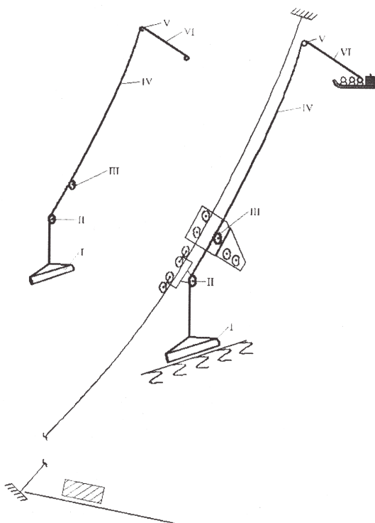
ნახ. 1. ა, ბ – განივგადასატანი საბაგირო მორსათრევი დანადგარის კვლევის სქემა: ა – ურიკის ბლოკის ჩამჭერში დასაფიქსირებლად მორის ვერტიკალურად გადაადგილების ტრასა; ბ – ტრასაზე განლაგებული წინააღმდეგობის ძალების I-VI მოდების ნერტილები
