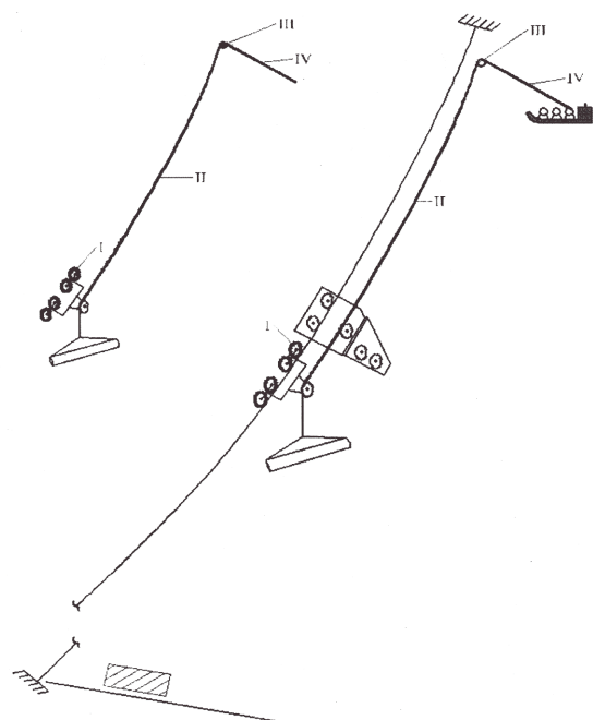
ნახ. 1. ა, ბ – განივგადასატანი საბაგირო მორსათრევი დანადგარის კვლევის სქემა: ა – ურიკის ბლოკის ჩამჭერში დასაფიქსირებლად მორის ვერტიკალურად გადაადგილების ტრასა; ბ – ტრასაზე განლაგებული წინააღმდეგობის ძალების I-VI მოდების ნერტილები
