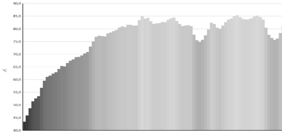
ნახ. 3. ცხელი ნარევის ტემპერატურის ცვლილება ორმოს ცენტრიდან საგზაო საფარის საზღვრამდე, რომელიც დამოკიდებულია ზედაპირის ფორმაზე ნარევის საფართთან კონტაქტისას :
