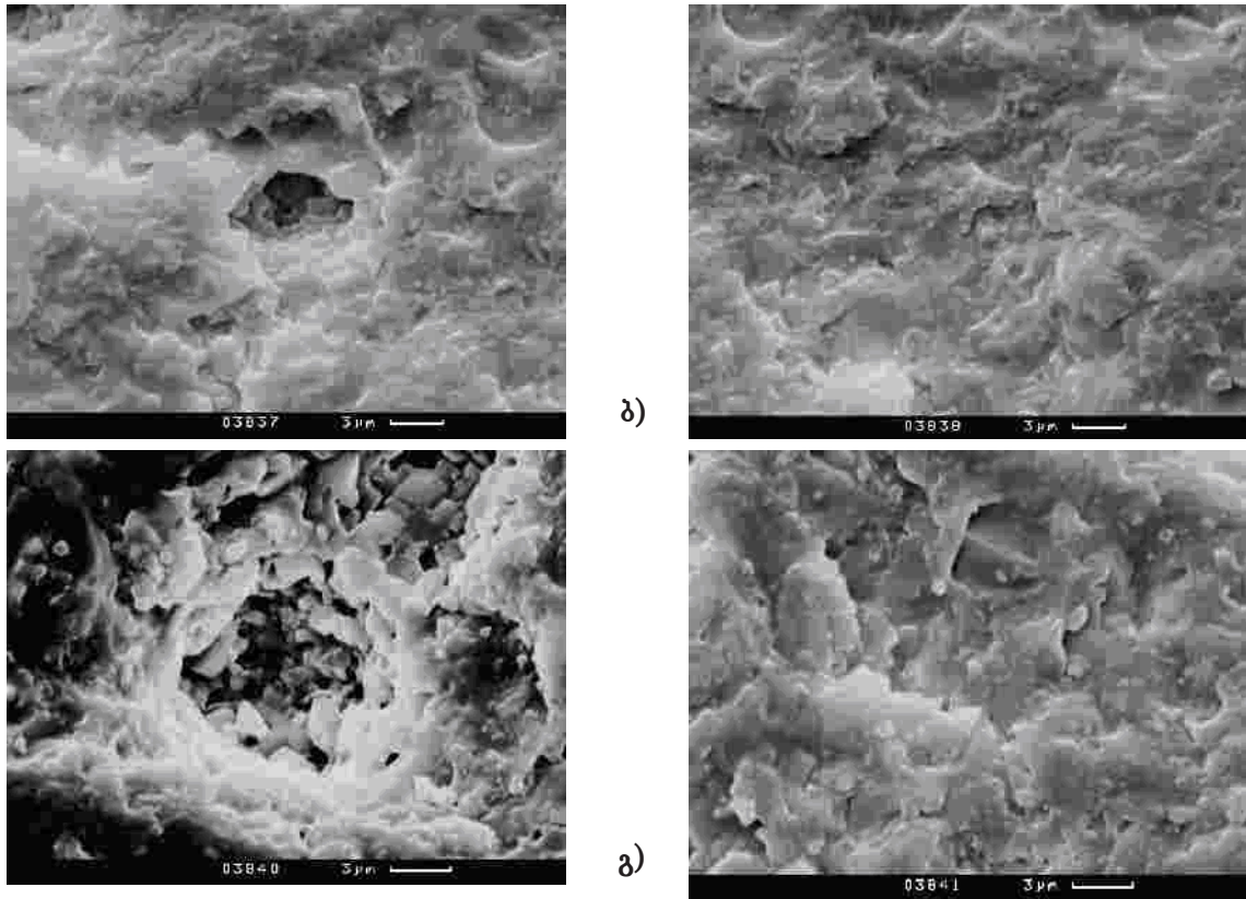
სურ.5. C 8 მასალის ელექტრონულ – მიკროსკოპიული სურათები გამომწვარი: ა)1400°C; ბ)1430°C; გ)1470°C X 4000.
