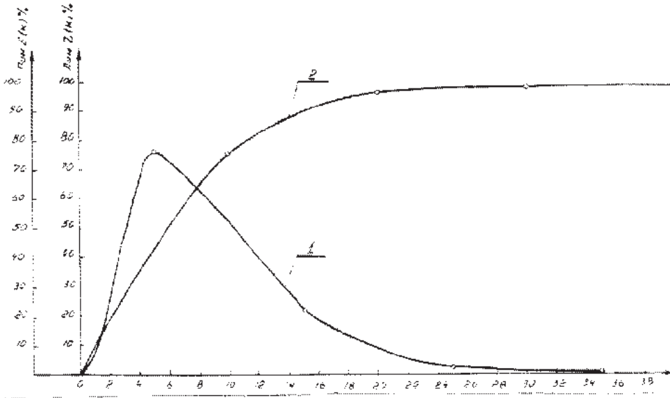
სურ.7. C 8 კერამიკის დახურული ფორიანობის ხაზობრივი ანალიზი: 1 – ფორების სიხშირე; 2 – ფორიანობის ჯამური სიხშირე.
