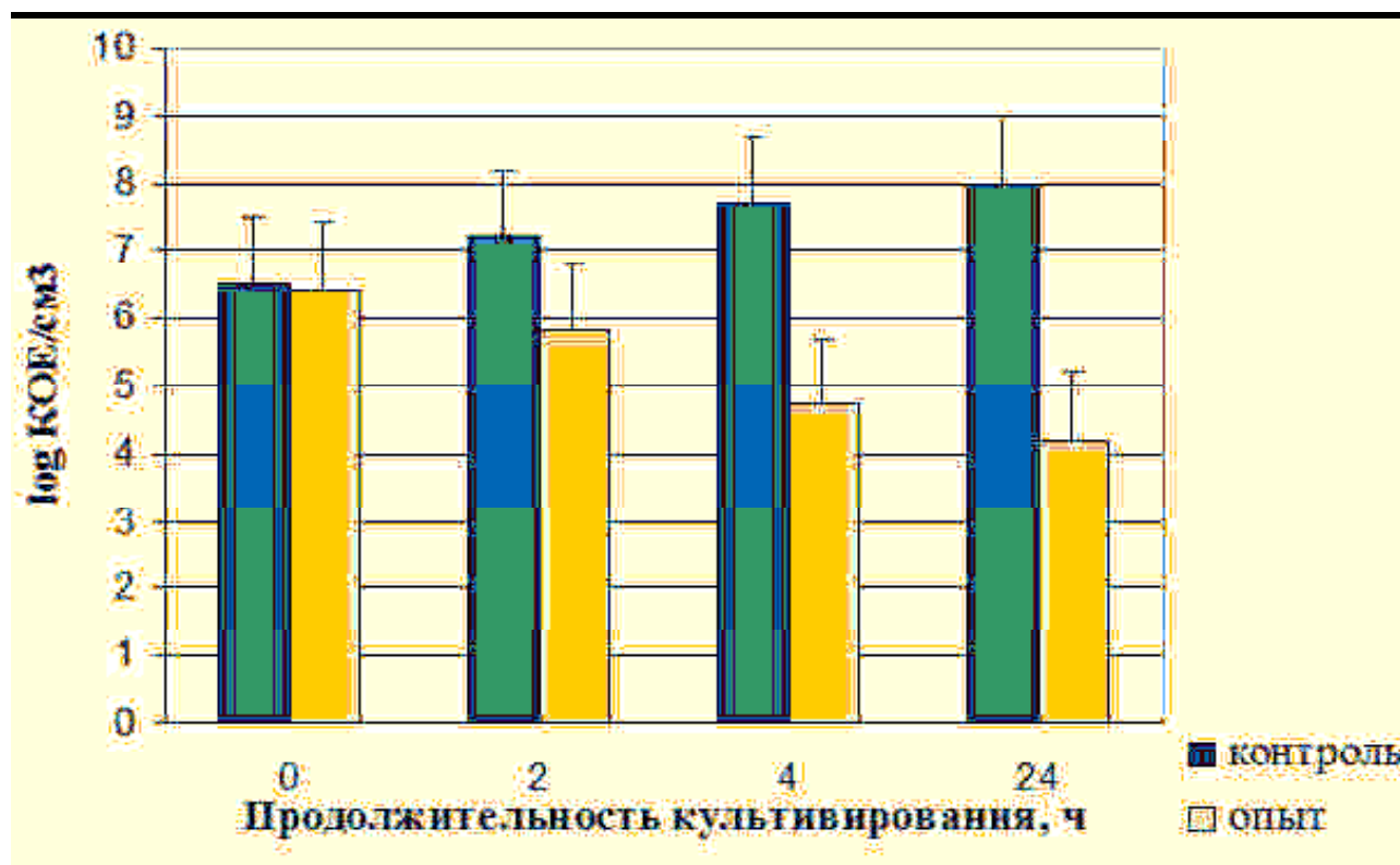
Рисунок 3– Влияние микрофлоры кисломолочного напитка на развитие и E.coli в процессе культивирования
