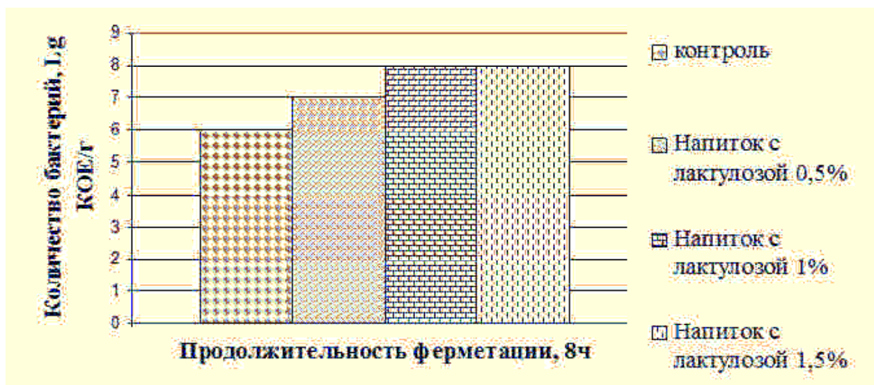
Рисунок 2 - Зависимость количества жизнеспособных молочнокислых бактерий в зависимости от количества внесения сиропа лактулозы
