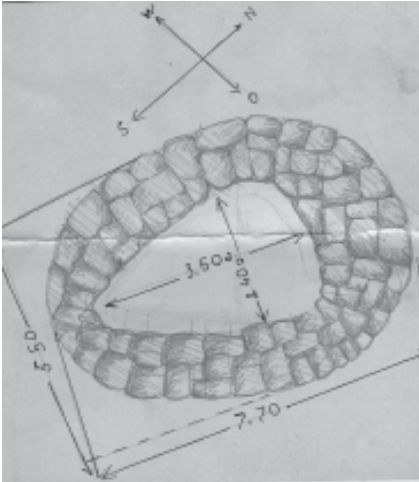
თამარის ციხე კოშკის ზედხედი
