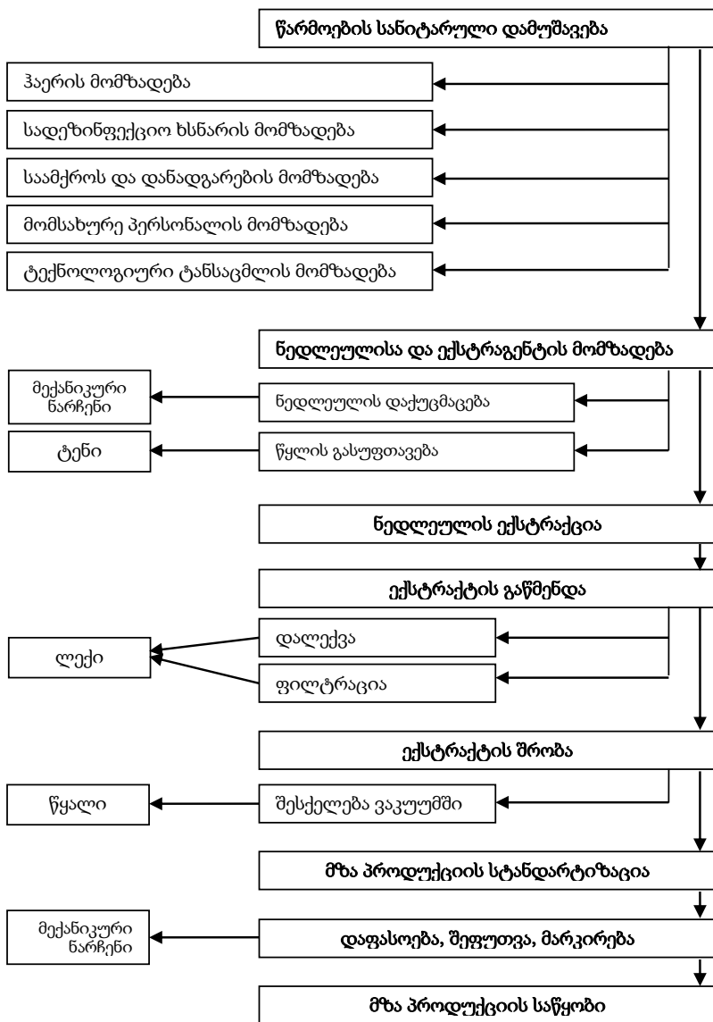
ნახ.1. ჩაის ფოთლის კატექინების კომპლექსის მიღების ტექნოლოგიური სქემა
