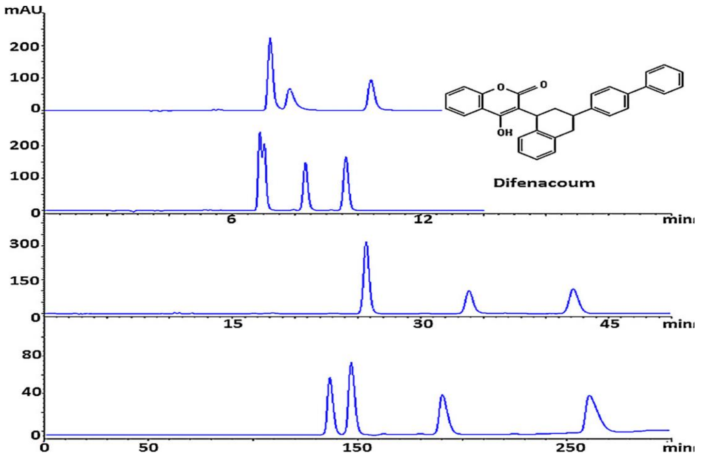
სურათი 14. დიფენაკუმის ენანტიომერების დაყოფა Lux ცელულოზა-1 აცეტონიტრილში (a), აცეტონიტრილ-წყალი (90/10, v/v) (b), აცეტონიტრილ-წყალი (70/30, v/v) (c), და აცეტონიტრილ-წყალი (50/50, v/v) (d), მობილური ფაზები. ყველა შემთხვევაში მობილური ფაზა შეიცავდა 0.1% ჭიანჭველმკვასს.
