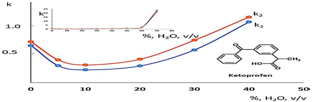
სურათი 10. აცეტონიტრილში წყლის შემცველობაზე დამყარებული შეკავება Lux ამილოზა - 2 სვეტზე.
