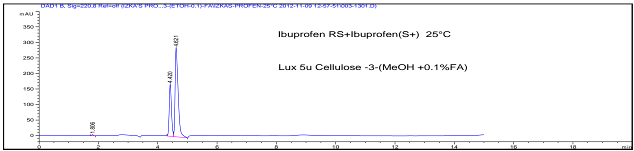
სურათი 3. იბუპროფენის დაყოფა ცელულოზა - 3 სვეტზე მოძრავ ფაზად მეთანოლის გამოყენებით
