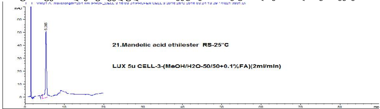
სურათი 4. ნუშის მჟავის დაყოფა ცელულოზა-3 სვეტზე, მოძრავ ფაზად მეთანოლის გამოყენებით
