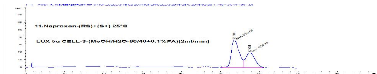
სურათი 5. ნაპროქსენის დაყოფა ცელულოზა-3 სვეტზე, მოძრავ ფაზად მეთანოლის გამოყენებით
