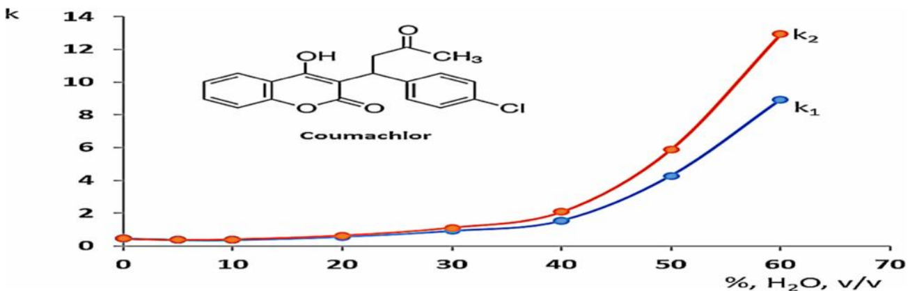
სურათი 6. კოუმაქლორის ენანტიომერების მეთანოლში წყლის შემცველობაზე დამყარებული შეკავების დროის დამოკიდებულება Lux ცელულოზა - 3 სვეტზე მრუდების გაყოფა ხდება მოძრავ ფაზაში წყლის მაღალი შემცველობისას, რაც ძირითადად ადასტურებს ენანტიომერების დაყოფის დაწყებას. მობილურ ფაზაში წყლის მოცულობის გაზრდით,
