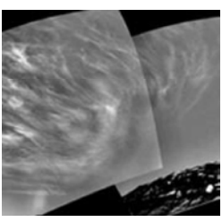
Тем временем ровер Opportunity передал изображение облаков, поразительно похожих на перистые облака Земли.
