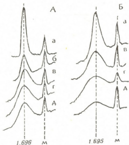
Рис. 6. Распределение ДНК хлоропластов в градиенте плотности CsCl. А — Sp. oleracea , Б — P. sativum . а — нативная, б — фрагментированная с помощью капилляра, в, г, д — фрагментированная с помощью ультразвука; время фрагментации 3,5 и 10 мин соответственно
