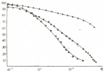
Рис. 5. Кинетика реассоциации ДНК в 1,0 \times SSC . \Delta — основной компонент, \bullet — сателлитный компонент, \blacksquare — ДНК фага T2
