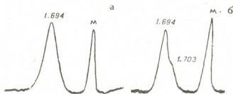
Рис. 1. Распределение ядерных ДНК в градиенте плотности CsCl. а— Ph. aureus , б— Ph. vulgaris , М—ДНК M. lysodeikticus
