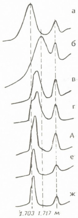
Рис. 4. Распределение спутникового компонента ДНК Ph. vulgaris в градиенте плотности CsCl . а—нативный, б—денатурированный. Далее ренатурированные при разных значениях C_0t , в—0.03, г—0.12, д—1.44, е—3.0, ж—16.0
