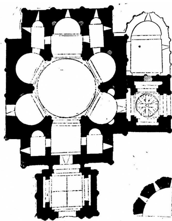
სურ. 104. ნიკორწმინდას ტაძარი. 1010—1014 წწ. გეგმა. ანაზომი 5. სევეროვსა.
