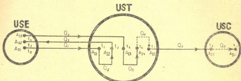
Рис. 1. Пример схемы подсистем USE , UST и USC глобальной системы операций.
