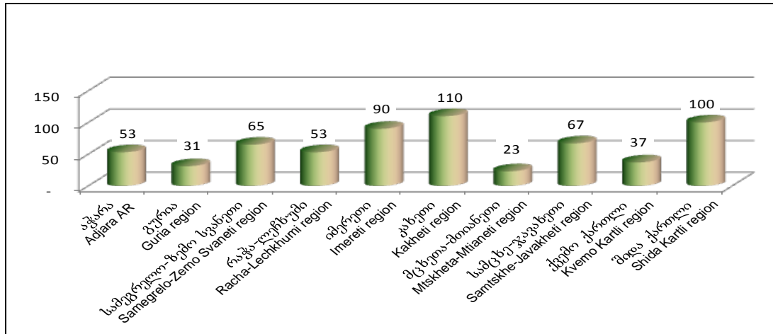
ნახ.6. ხეტყის ნარჩენი ბიომასა საქართველოს რეგიონებისათვის (ათასი მ 3 )
