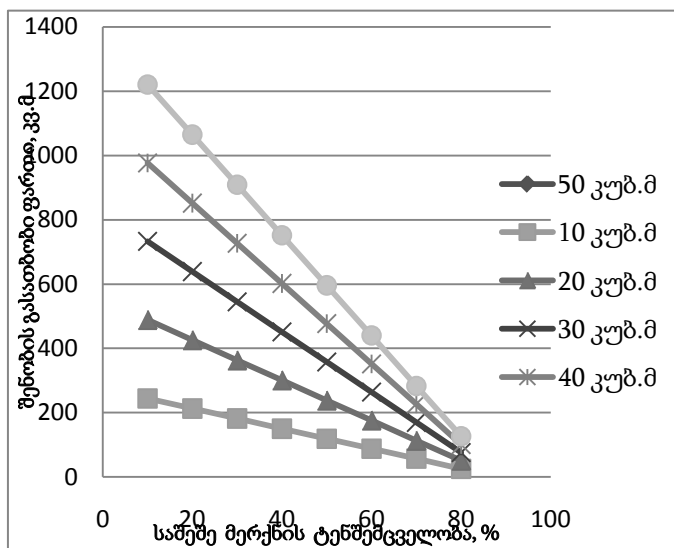
ნახ.3. შენობის გასათბობი ფართის დამოკიდებულება საშეშე მერქნის ტენშემცველობაზე
