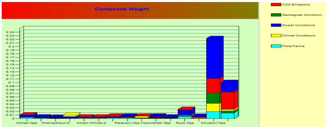
ნახ. 6. თითოეული ჰესის გარემოზე ზემოქმედების დონე
