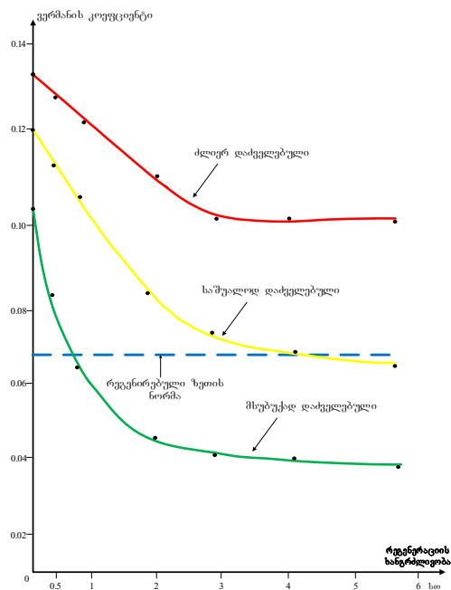
ნახ. 6 20% გუმბრინის თიხით რეგენირებული ზეთების ვერმანის კოეფიციენტის დამოკიდებულება რეგენერაციის ხანგრძლივობაზე.
