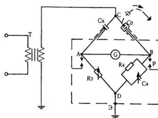
ნახ №1 ტრანსფორმატორის ზეთის დიელექტრიკული დანაკარგების და შეღწევადობის შერინგის ბოგირით გაზომვის გამარტივებული სქემა.
