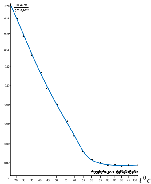
ნახ. 3 გუმბრინის თიხით რეგენირებული ზეთის მჟავური რიცხვის დამოკიდებულება რეგენერაციის ტემპერატურაზე.
