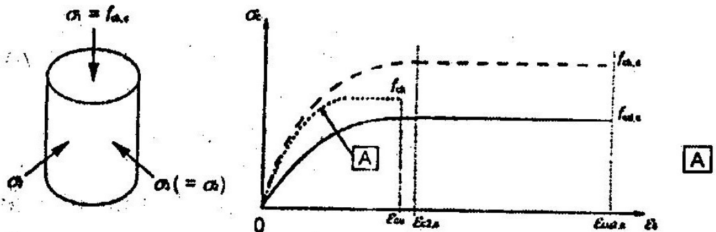
ნახ.14. დამოკიდებულება "ძაბვა-დეფორმაცია" შორის შეზღუდული ბეტონისათვის.
