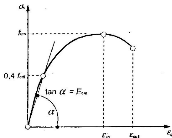
ნახ.10. კონსტრუქციების გაანგარიშებისას სქემატური თანაფარდობა
