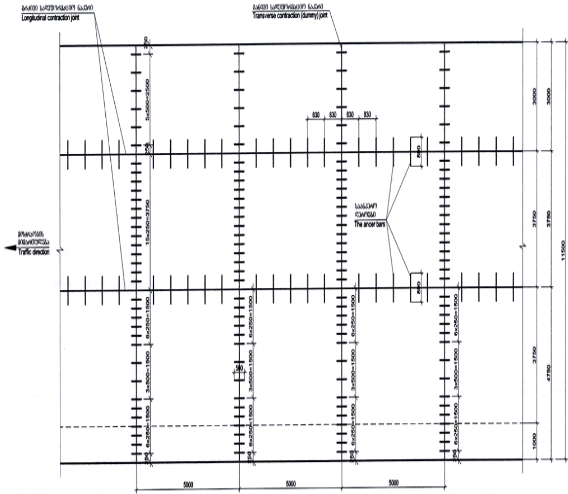
ნახ. 8. შეკუმშვისა და გაფართოების ნაკერების სქემა ცემენტობეტონის საგზაო ფილაში: 1-გაფართოების ნაკერი; 2- შეკუმშვის ნაკერი; 3-გრძივი ნაკერი; 4- ფილა.
