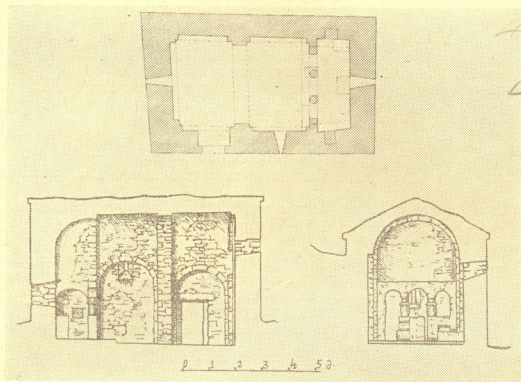
Рис. 3. Адцрисхеви. План, разрез на юг и разрез на восток
