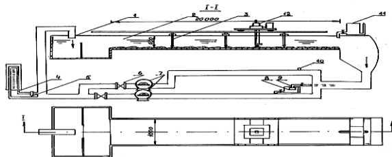
ნახ. 2. ექსპერიმენტული დანადგარი
