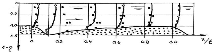
ნახ. 3 მდინარეში ფსკერულ წარმონაქმნებზე გასაშუალოებული \phi და პულსაციურ - • სინქარეთა განაწილების ეპიურები.
