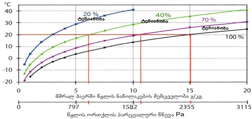
ნახ. 1. წყლის ორთქლის რაოდენობის განსაზღვრა მშრალ ჰაერში გ/კგ
