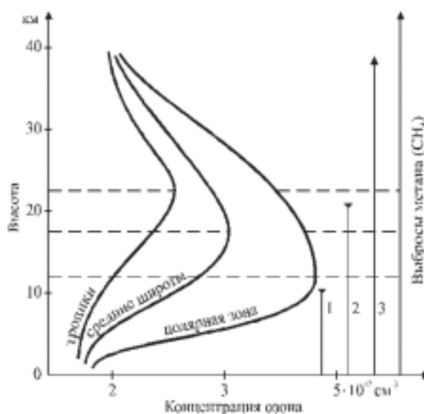
Рис. 10. Широтное распределение озона и техногенно-природные источники метана:
