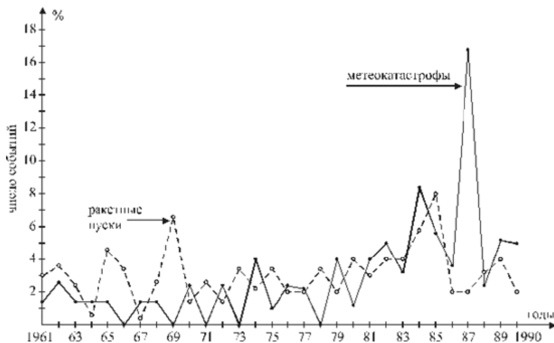
Рис. 8. Распределение количества ракетных пилотируемых пусков ( n = 132 ) и метеокатастроф ( n = 68 ) по годам (1961-1990 гг.).
