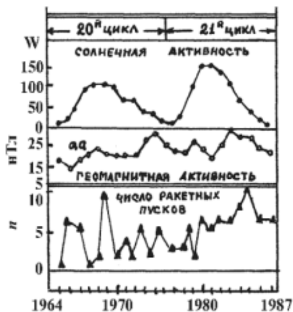
Рис. 9. Гелиофизическая (W) и геомагнитная (aa) обстановки в годы активности пусков пилотируемых космических аппаратов (n — число пусков)
