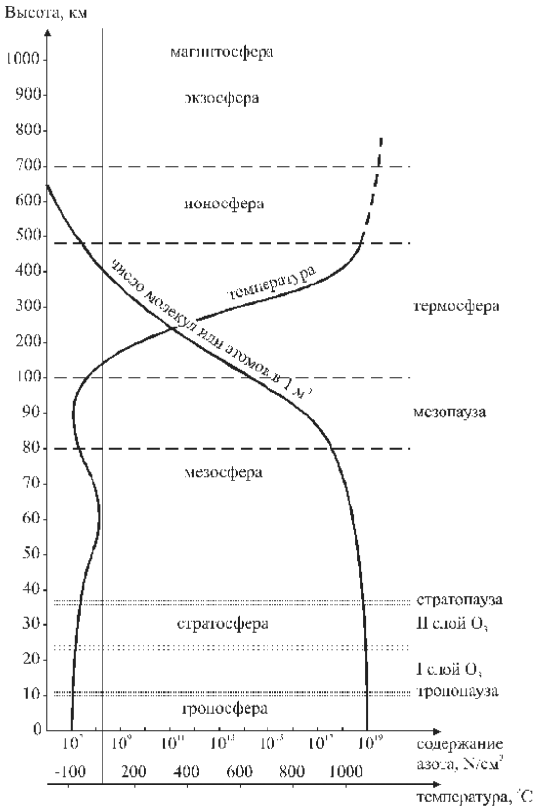
Рис. 2. Общая схема строения нижнего геокосмоса
