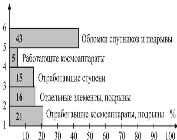
Рис. 7. Состав космического мусора ракетного происхождения
