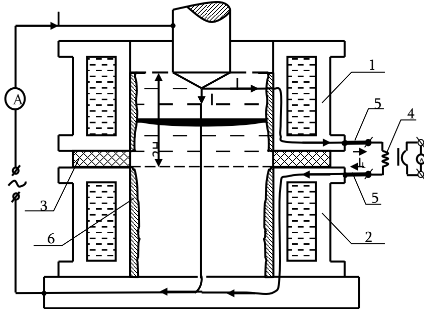
ნახ. 2. დაშუნტვის დენის გაზომვის სქემა. 1-2-ზედა და ქვედა კრისტალიზატორი; 3-საიზოლაციო ფენა; 4-დენის ტრანსფორმატორი; 5-დენმიმყვანი სადენები; 6-წიდის ქერქი.
