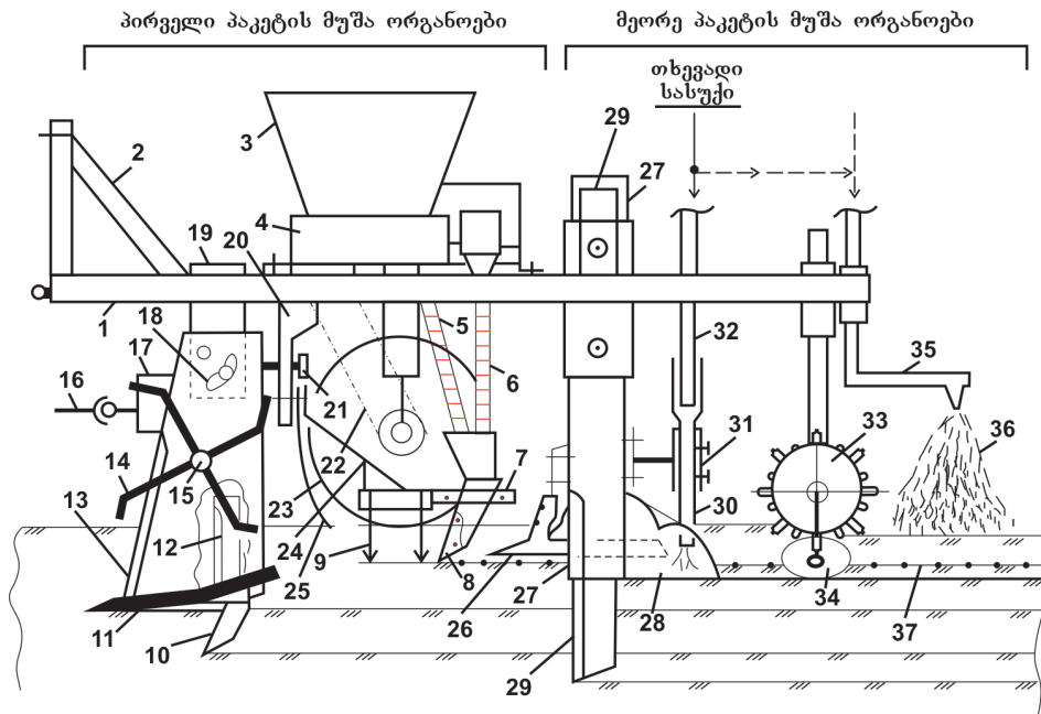
ნახ. 1. ნიადაგის ზოლურად სახნავ-სათესი და მცენარეთა მოვლის პაკეტურ-კომბინირებული მანქანის სქემა. პირველი პაკეტის მუშა ორგანოები: 1-ჩარჩო; 2-საკიდარი; 3-თესლისა და სასუქის სათავსი; 4-თესლისა და სასუქის გამომთესი მოწყობილობა; 5-სასუქის მილგამტარი; 6-თესლის მილგამტარი; 7-ჩამთესის სამაგრი კრონშტეინი; 8-ანკერული ჩამთესი; 9-კბილებიანი ფარცხი; 10-ნიადაგამღრმავებელი; 11-მთავარი სახნისი (სოლი); 12-გვერდითი გამაფართოებელი ირიბი დანები; 13-გვერდითი ვერტიკალური დანები; 14-ფრეზის დანები; 15-ფრეზის ლილევი; 16-კარდანული გადაცემა; 17-ფრეზის ამძრავი რედუქტორი; 18-მთავარი სახნისის ნიადაგში შეჭრის კუთხის სარეგულირებელი ქანჩი ოვალური ღარით; 19-სახნავი ორგანოს ჩარჩოზე სამაგრი კრონშტეინი; 20-კრონშტეინი; 21-საყრდენი ქანჩი; 22-სათესი მოწყობილობის ამძრავი ჯაჭვი; 23-საყრდენ-სარეგულირებელი თვალი; 24-ფარცხისა და ჩამთესის (8) სამაგრი კრონშტეინი; 25-ბელტის (გოროხების) გატყორცვის შემზღვეველი ბადე. მეორე პაკეტის მუშა ორგანოები: 26-კულტივატორის უნივერსალური ისრისებური თათი; 27-მინი სარწყავი არხების გამჭრელი დანა, ფრით (28); 29-დარმჭრელი-მიმართველი დანა; 30-თხევადი სასუქის ლითონის მილგამტარი; 31-სამაგრი კრონშტეინი; 32-თხევადი სასუქის რეზინის მილგამტარი; 33-წემისებურ-კბილანური სამსხვრევ-სატკეპნი საგორავი; 34-სატკეპნი საგორავი (ან ციგისებური შემზღვეველი ფარი); 35-სასხურებლის შტანგა; 36-შხამ-ქიმიკატი; 37-თესლი (სასუქი).
