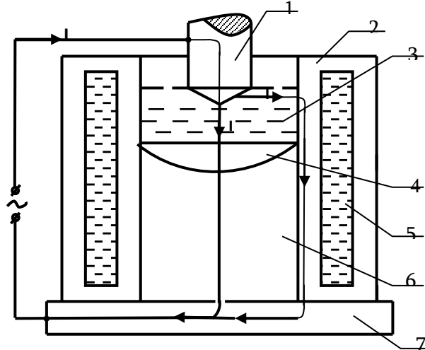
ნახ.1. ლითონების ელექტროქიმიური გადადნობის და დენის გავლის სქემა. 1-გადასადნობი ელექტროდი; 2-კრისტალიზატორის შიგა კედელი; 3-გამდნარი წიდა; 4-გამდნარი ლითონის აბაზანა; 5- წყალი; 6- ლითონის სხმული ; 7-კრისტალიზატორის ძირი. I -გადადნობის სრული დენი; I_w -წიდაში გამავალი ძირითადი დენი; I_L -კრისტალიზატორის კედელში გამავალი დაშუნტვის დენი.
