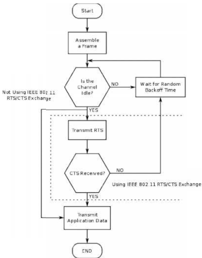
ნახ. 2. ტექნოლოგია CSMA/CA.
