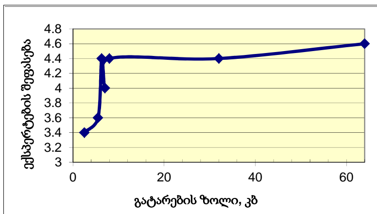
ნახ. 3 კავშირის ხარისხის დამოკიდებულება გატარების არხის სიგანეზე (დიაპაზონი)
