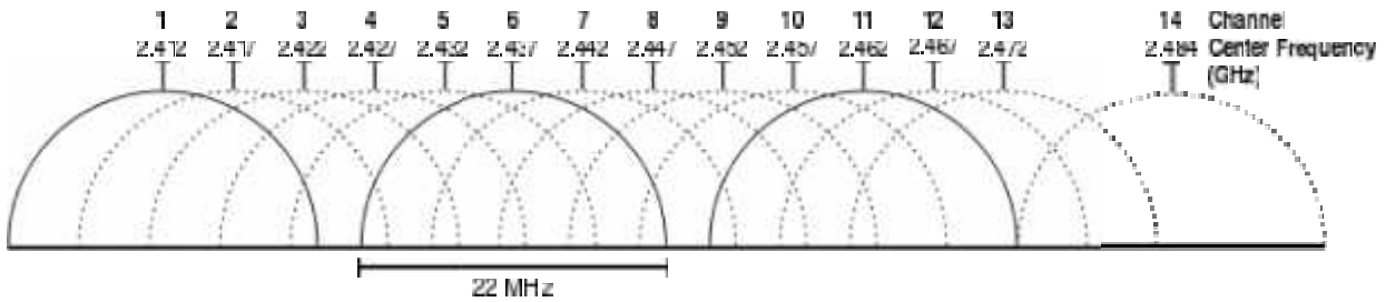
ნახ. 1. არხების დიაპაზონები და მათი განაწილების სქემა
