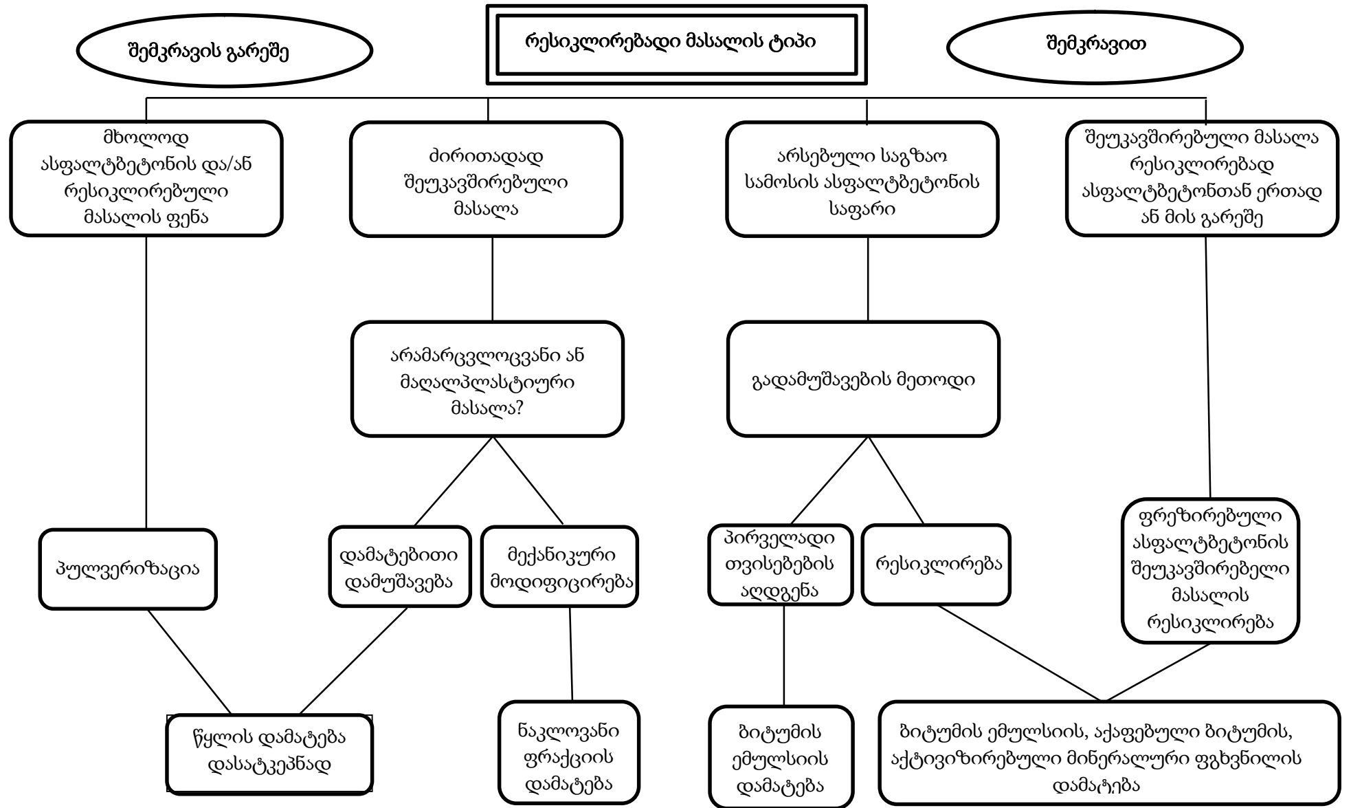
ნახ.1. ასფალტბეტონის დაზიანებული საფარის რესიკლირების ტიპები
