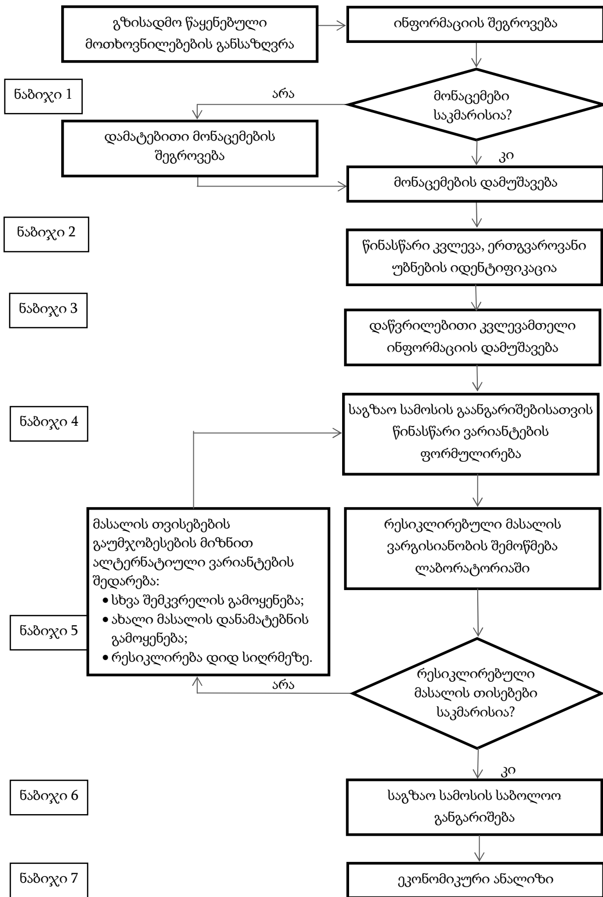
ნახ. 2. საგზაო სამოსის კვლევა და გაანგარიშება. ბლოკ-სქემა
