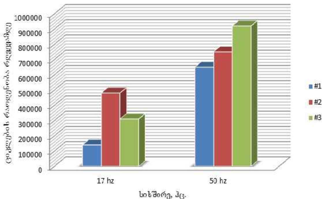
ნახ. 1. ასფალტბეტონების დალილობითი ხანგამძლეობა დატვირთვის სხვადასხვა სიხშირეებზე
