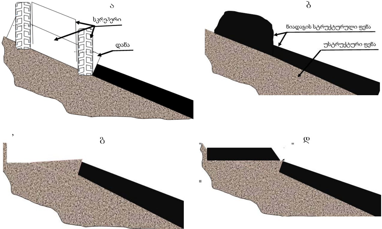
ნახ. 3. ქანობის ტერასირება ა – სკრეპერით სტრუქტურული ფენის მოჭრა, ბ – მოჭრილი ფენის მოგროვება, გ – უსტრუქტურო ფენისაგან ტერასის ჩამოყალიბება (შექმნა) და დ – ტერასზე სტრუქტურული ნიადაგის მოსწორება
