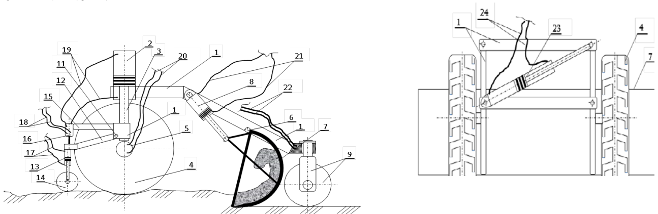
ნახ. 5. ავტომატური მართვის სისტემის მქონე სკრეპერის პრინციპული სქემა, გვერდხედში.
