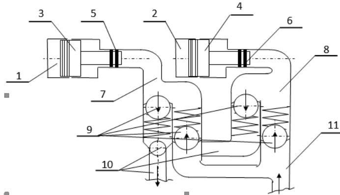
ნახ. 6. თავისუფალდგუშიანი შიგაწვის ძრავა 1, 2 – ცილინდრები, 3, 4 – დგუშები, 5, 6 – პლუნჟერები, 7, 8 – მილგამტარები, 9 – ავტომატური სარქველები, 10, 11 – მაგისტრარული მილგამტარები
