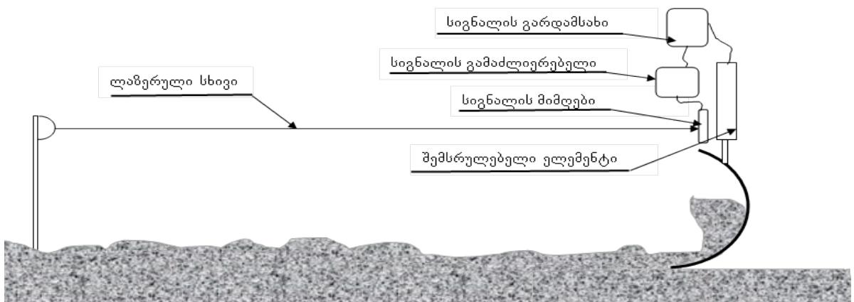
ნახ. 4. ლაზერული მართვის სისტემით მართვადი სამუშაო ორგანოს სქემა
