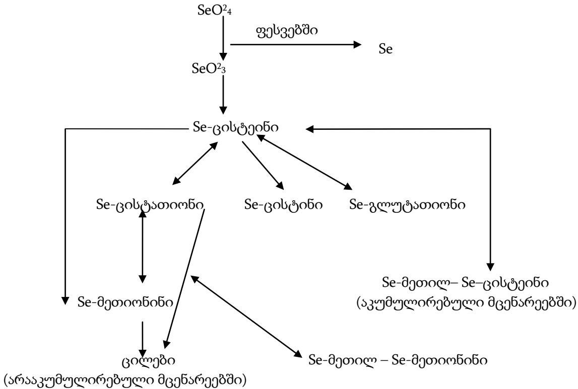
სქემა 1. სელენის მეტაბოლიზმი მცენარეებში
