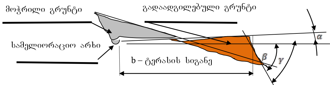
ნახ. 1. ტერასის წარმოქმნის ხერხი, \beta – ქანობის საწყისი დახრის კუთხე, \alpha – ტერასის დახრის კუთხე პორიზონტთან
