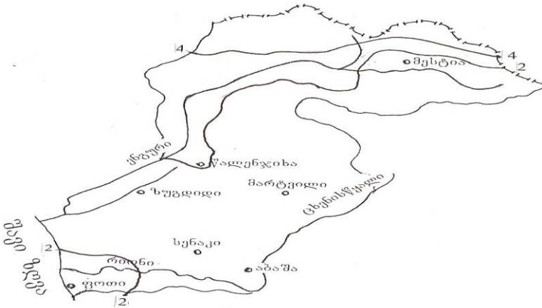
ნახ. 2.5.2. ქარის სიჩქარე. ივლისი. მ/წმ
