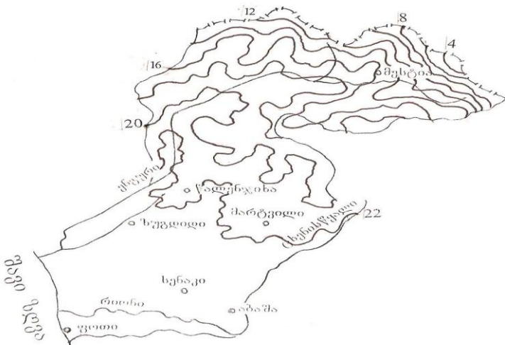
ნახ. 2.1.3. ჰაერის საშუალო თვიური ტემპერატურა . ივლისი.
