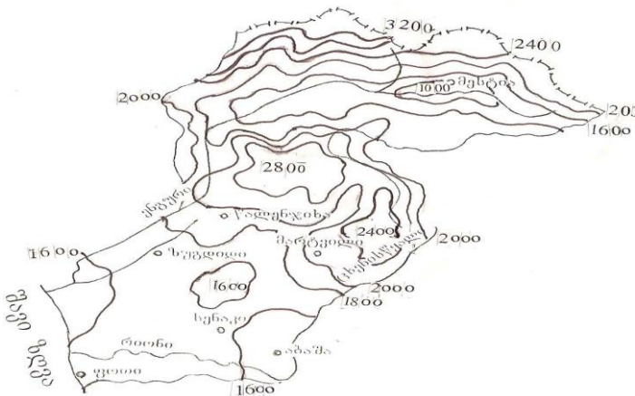
ნახ. 2.3.1. ატმოსფერული ნალექების წლიური ჯამები. მმ წლის ცივი პერიოდის განმავლობაში მოსული ნალექების ჯამი მერყეობს 400-1200მმ-ის ფარგლებში, ხოლო თბილი პერი-
