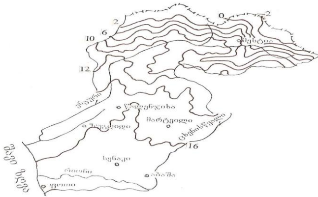
ნახ. 2.1.4. ჰაერის საშუალო თვიური ტემპერატურა . ოქტომბერი.
