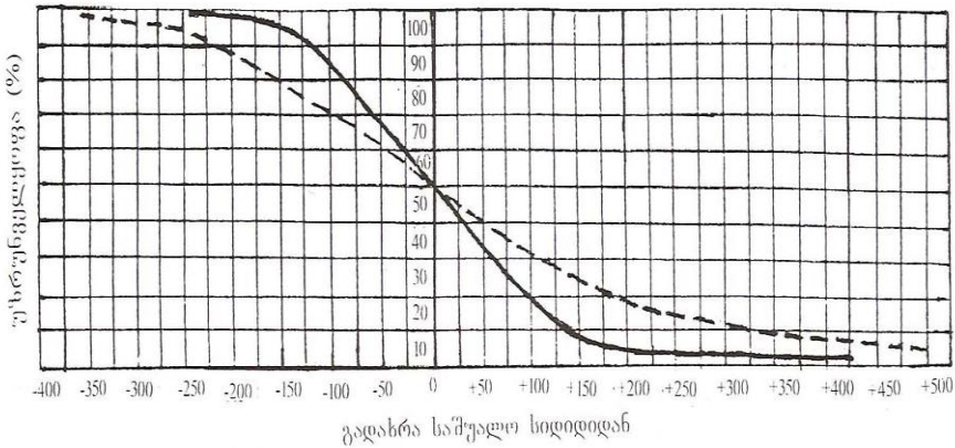
ნახ. 3.2.2. ნალექების უზრუნველყოფის მრუდი 10 0 -ზე ზევით ტემპერატურის პერიოდში -----ნალექების ჯამი ≥ 700 მმ ——— ნალექების ჯამი ≤ 700 მმ
