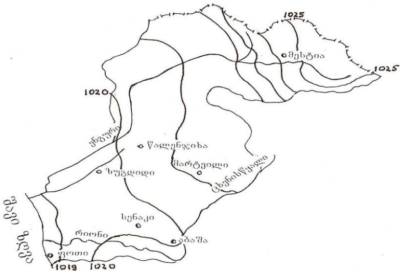
ნახ.1.2.1. ატმოსფერული წნევა. იანვარი. ჰჰა
