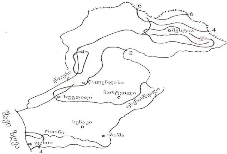
ნახ. 2.5.3. ქარის სიჩქარე. წელიწადი. მ/წმ
