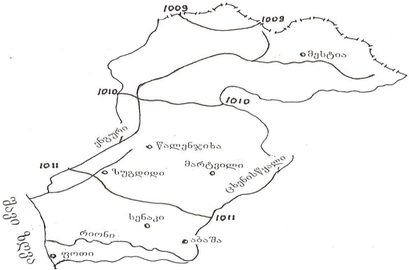
ნახ. 1.2.2. ატმოსფერული წნევა. ივლისი. კპა.
