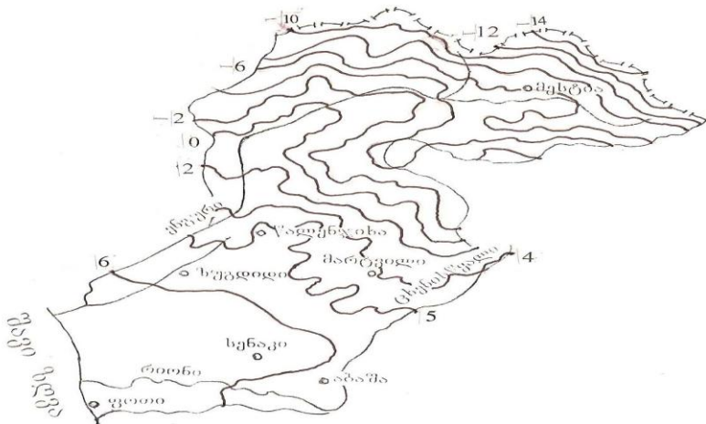
ნახ. 2.1.1. haeris saSualo Tviuri temperatura . ianvari.
