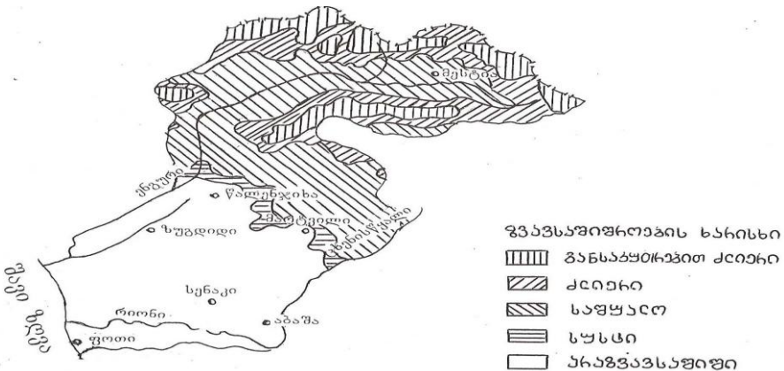
ნახ. 4.4.1. ზვავსაშიში რაიონები
