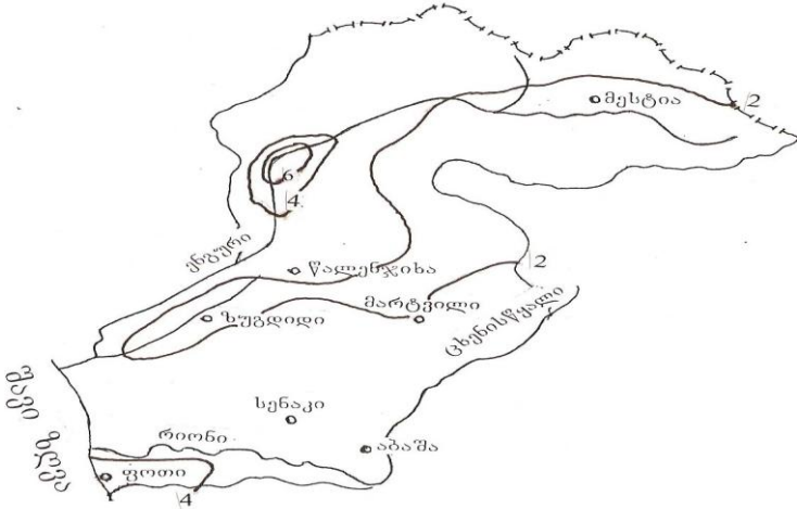
ნახ. 2.5.1. ქარის სიჩქარე. იანვარი. მ/წმ
