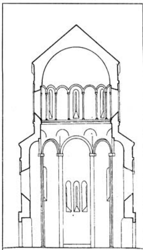
192. ნოჯიხევი. ეკლესიის რეკონსტრუქცია. განაკვეთი აღმოსავლეთით (არქ. რ. გვერდწითელის მიხედვით)
