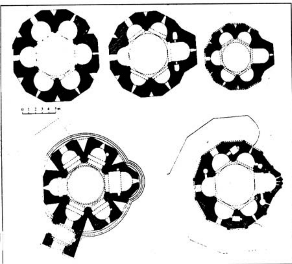
188. ექსავსიდა ანუ ეკლესიების ეკვებები: გოგეუბა, კაღმის-ალისი, ოღლისი, ბოჭორმა, კაცხი (ვ. ცინცაძის მიხედვით)
