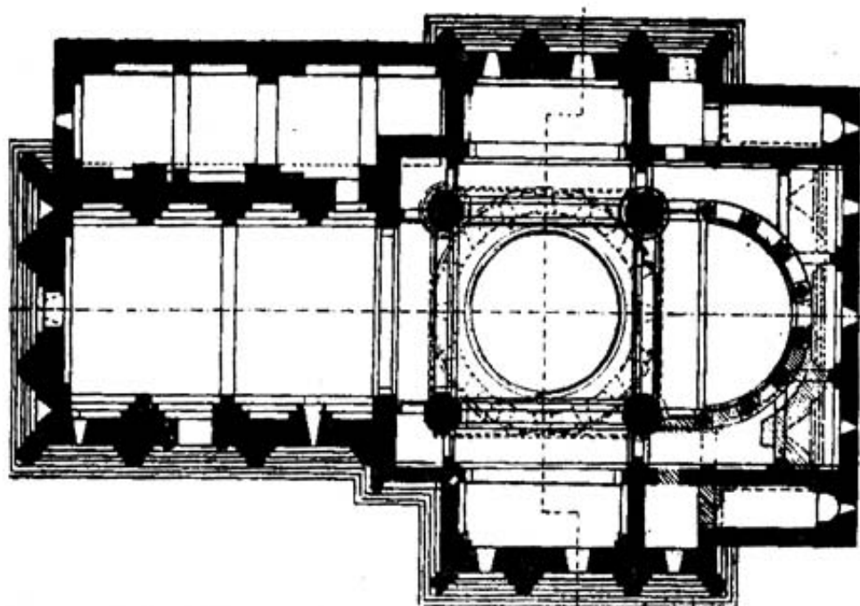
172. იშხანი. ტაძრის ვეგმა
