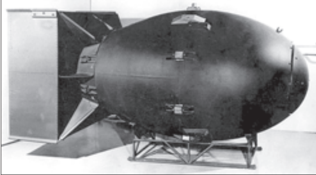
ნეიტრონული ბომბი
