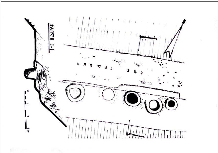
გალი, მზიური. რკინის ქურების გეგმა და ჭრილი
